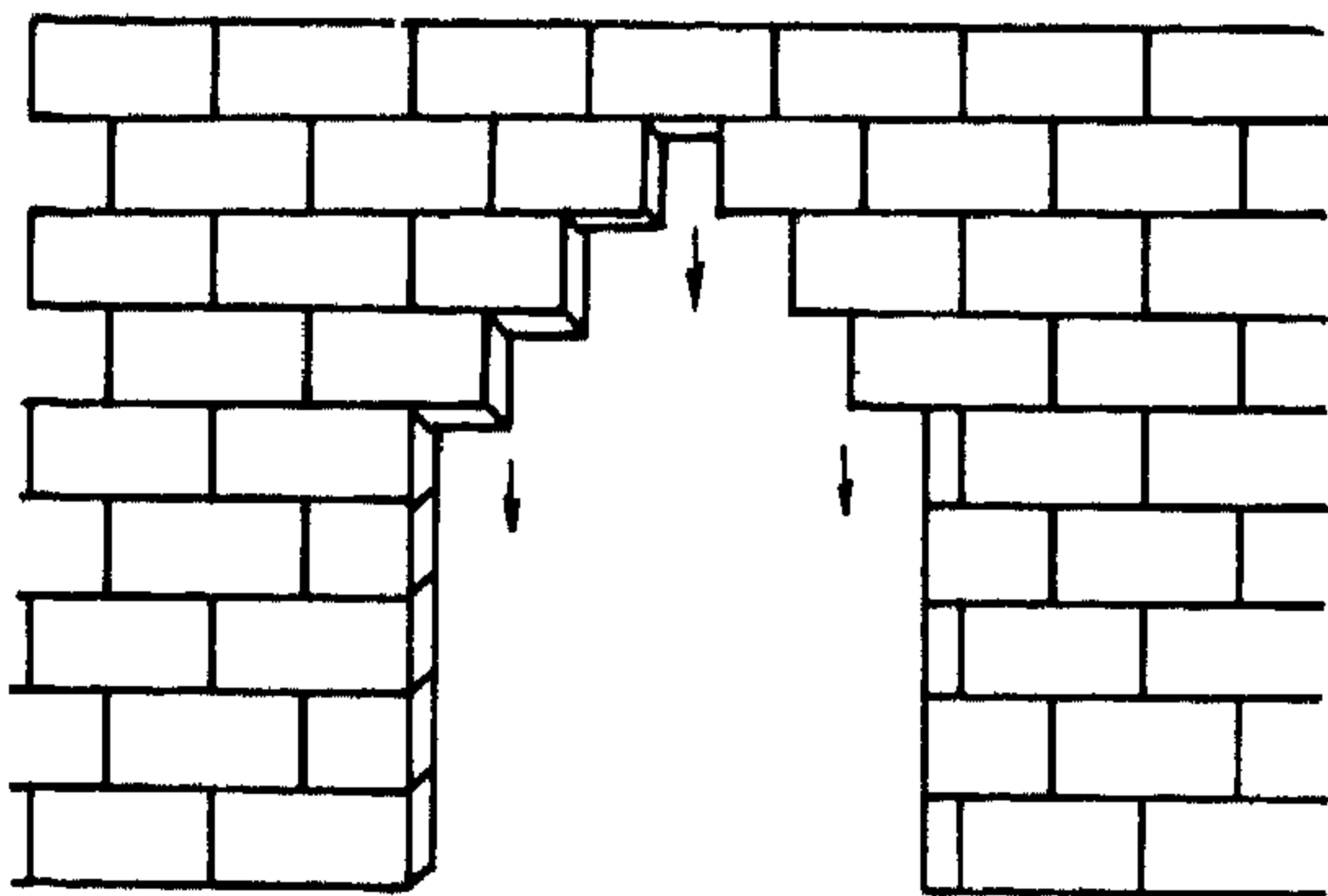
شكل (٦،٥) شكلان مختلفان لعقد مطنّف
